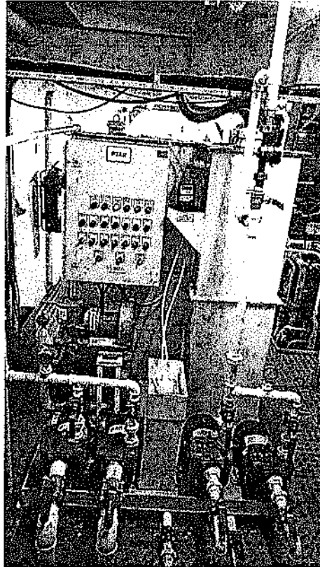
Fotografía No. 1 PTAR ubicada dentro de uno de los remolcadores
